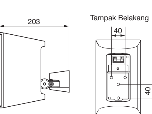
Tampak samping setelah dipasang pelengkap
