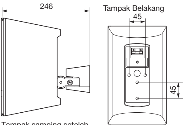
Tampak samping setelah dipasang pelengkap
